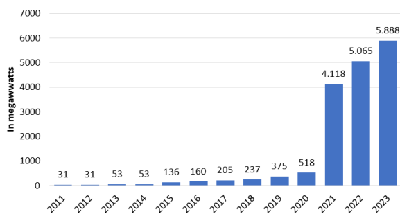
Biểu đồ 1. Tổng công suất năng lượng gió từ 2011 - 2023
